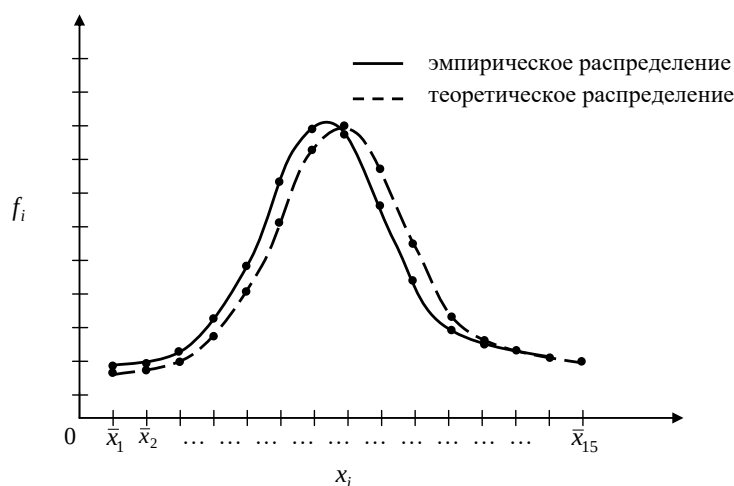
Рис. 1. График эмпирического и теоретического распределения
