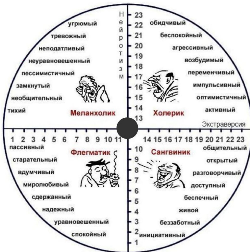
Рис. 1. Круг Айзенка.
