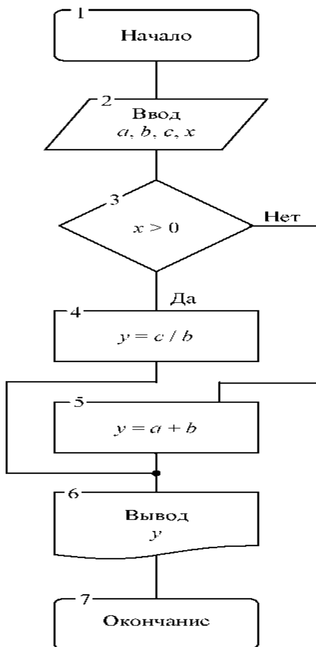
Рис. 3. Разветвляющийся алгоритм
